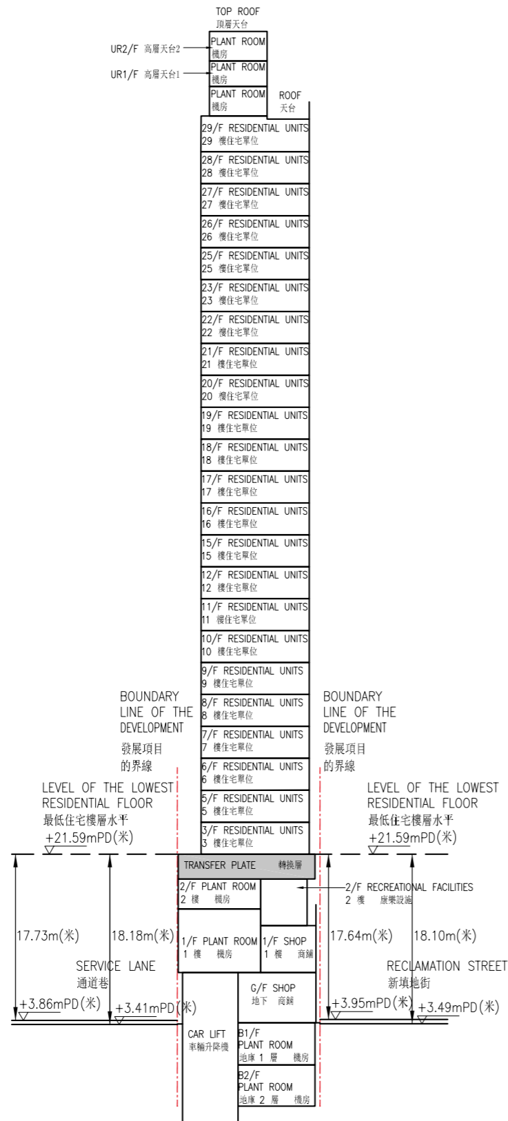
Cross-Section Plan 2 橫截面圖 2
